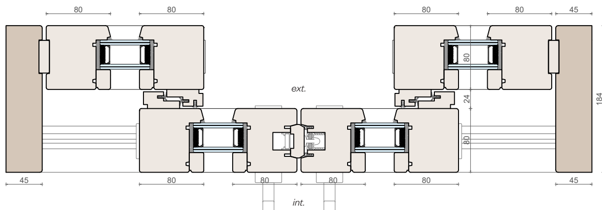
Sezione orizzontale
