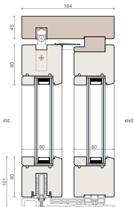
Sezione verticale
