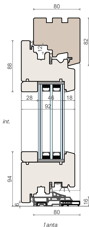
Sezione verticale
