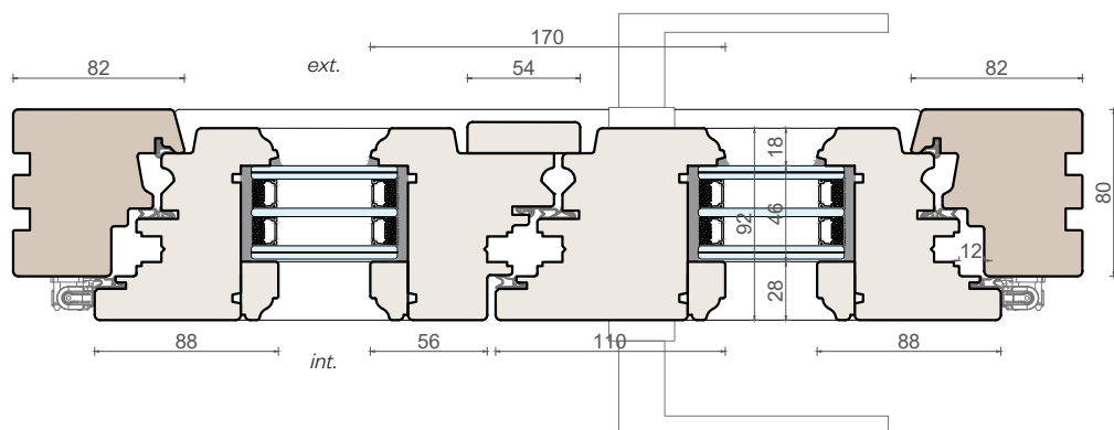
Sezione verticale
