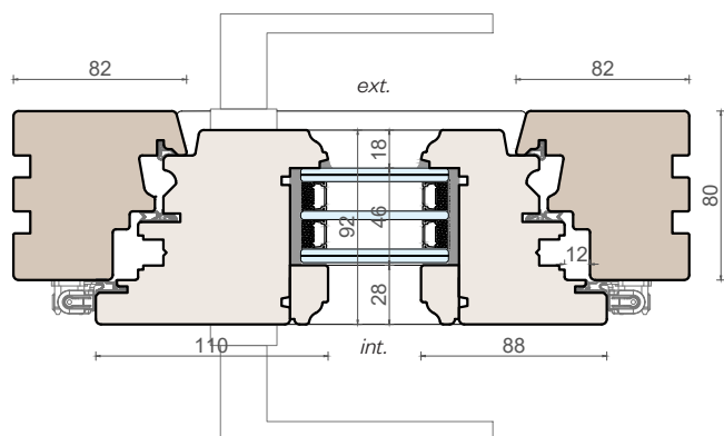
Sezione orizzontale
