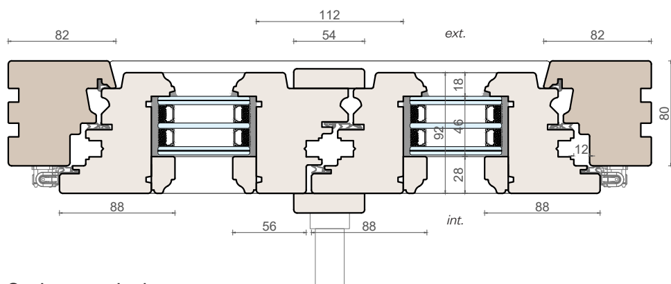
Sezione verticale
