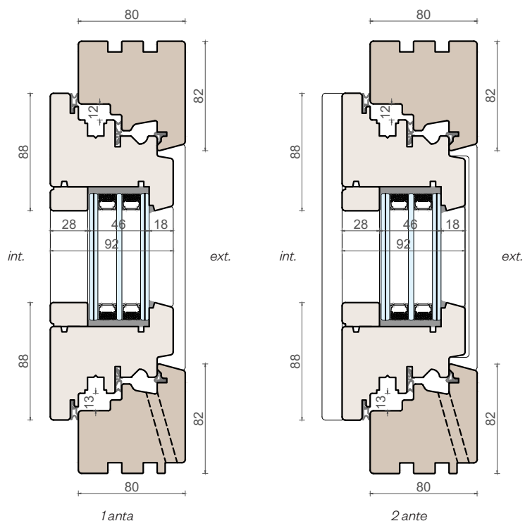
Sezione verticale
