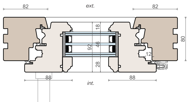
Sezione orizzontale
