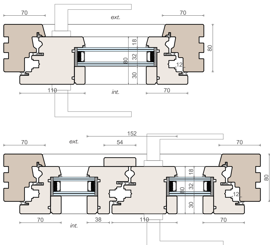
Sezione orizzontale
