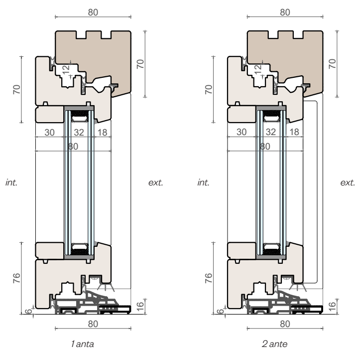
Sezione verticale
