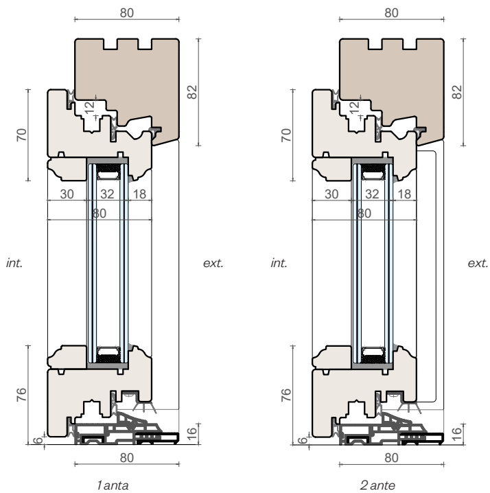
Sezione verticale
