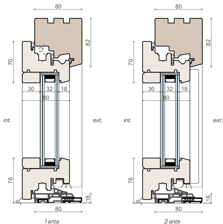
Sezione verticale
