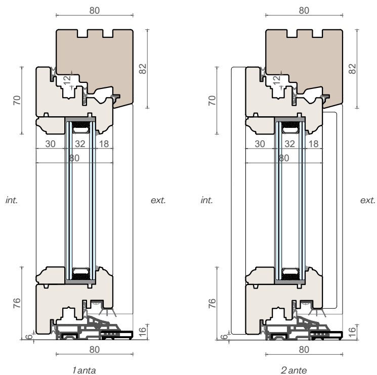
Sezione verticale
