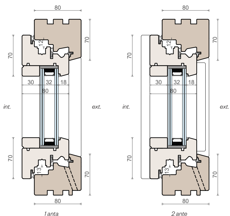
Sezione verticale
