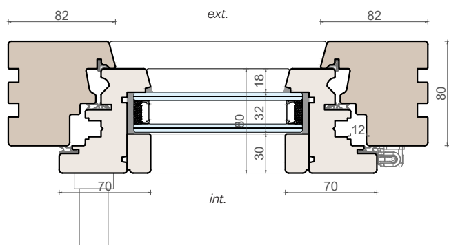
Sezione orizzontale
