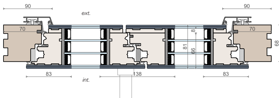
Sezione verticale
