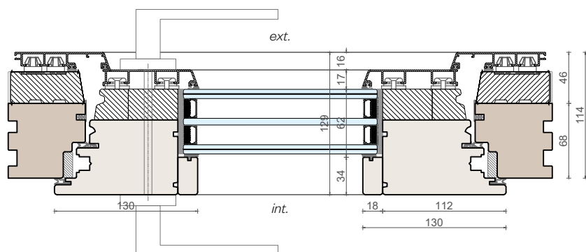
Sezione orizzontale
