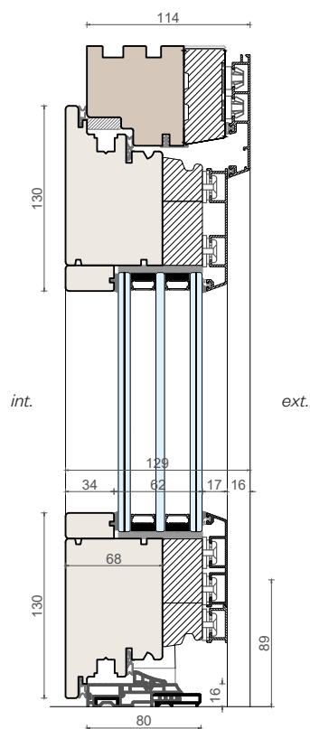
Sezione verticale
