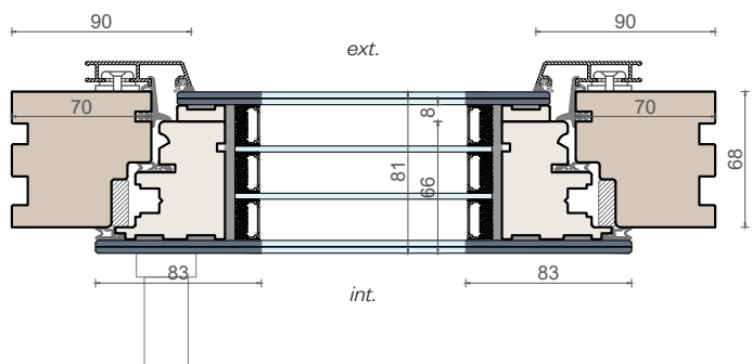
Sezione orizzontale
