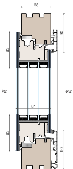
Sezione verticale
