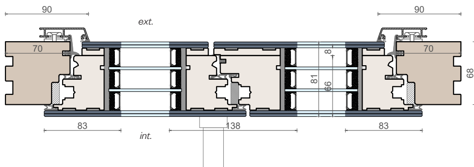
Sezione verticale
