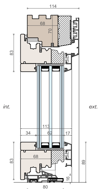
Sezione verticale
