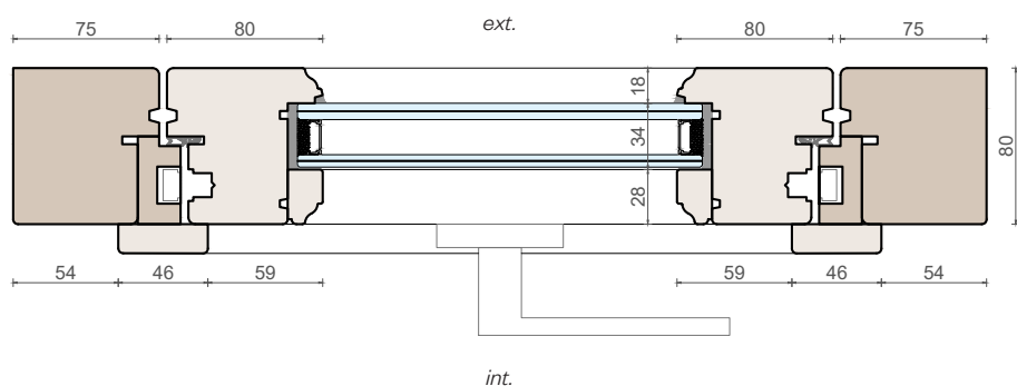
Sezione orizzontale
