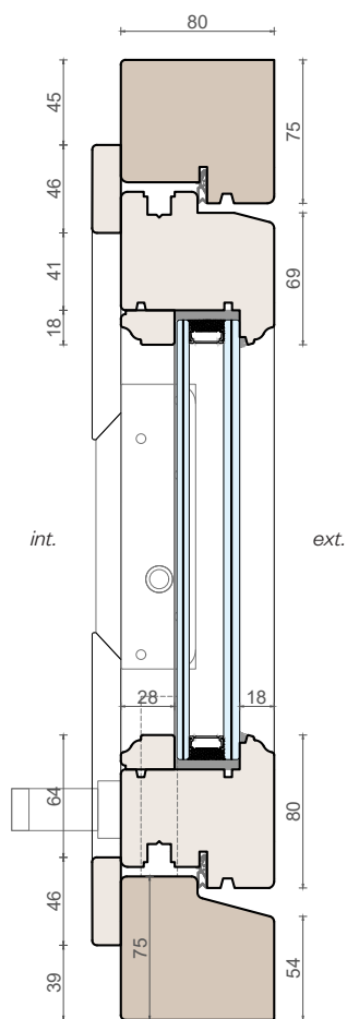
Sezione verticale
