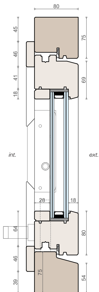
Sezione verticale
