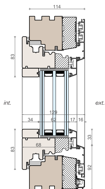
Sezione verticale
