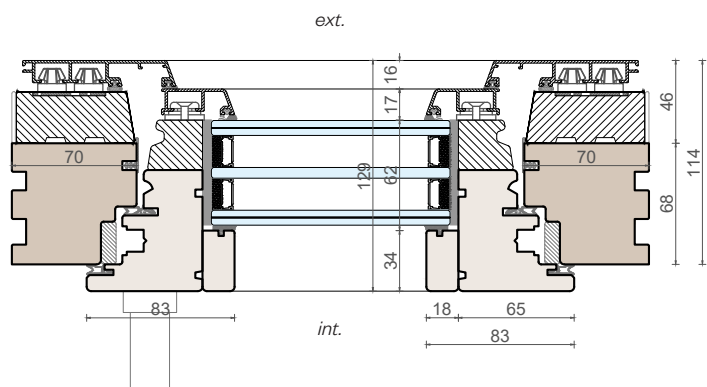
Sezione orizzontale
