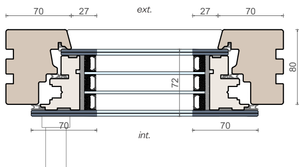
Sezione orizzontale
