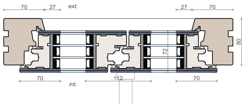
Sezione verticale
