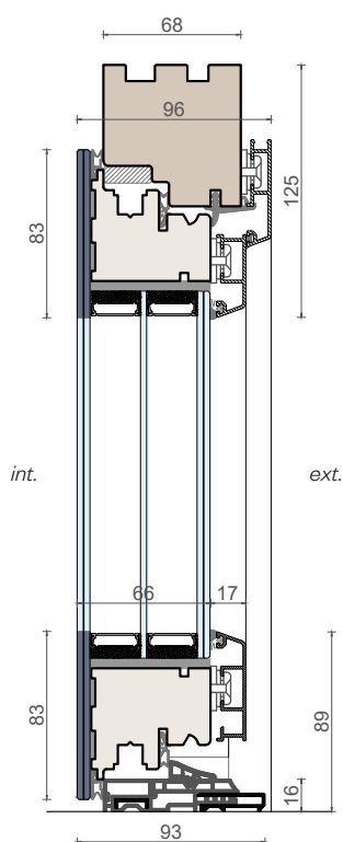
Sezione verticale
