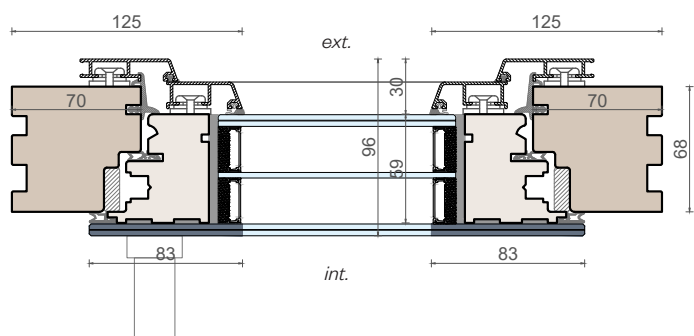
Sezione orizzontale
