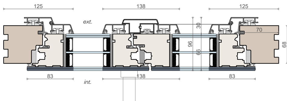
Sezione verticale
