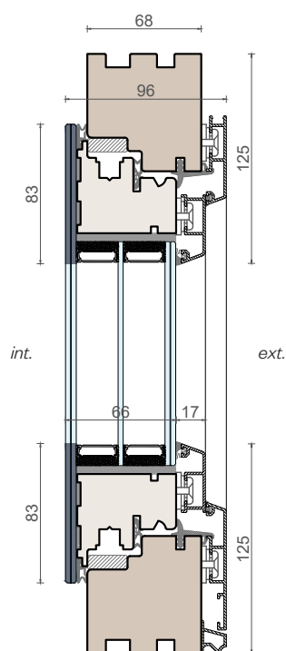
Sezione verticale
