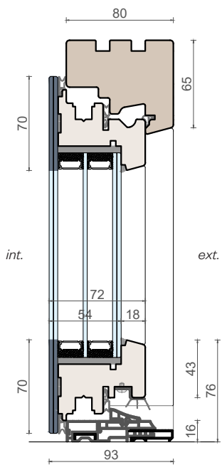
Sezione verticale
