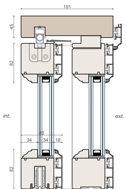
Sezione verticale
