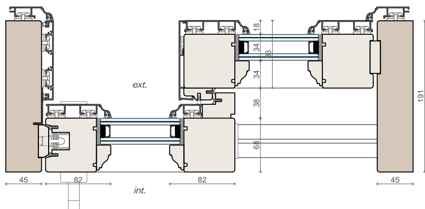
Sezione orizzontale - Versione Impero
