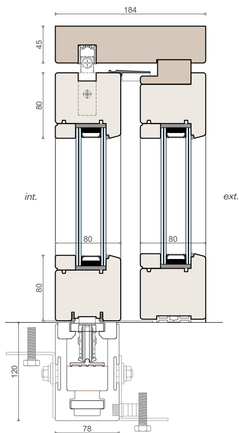
Sezione verticale
