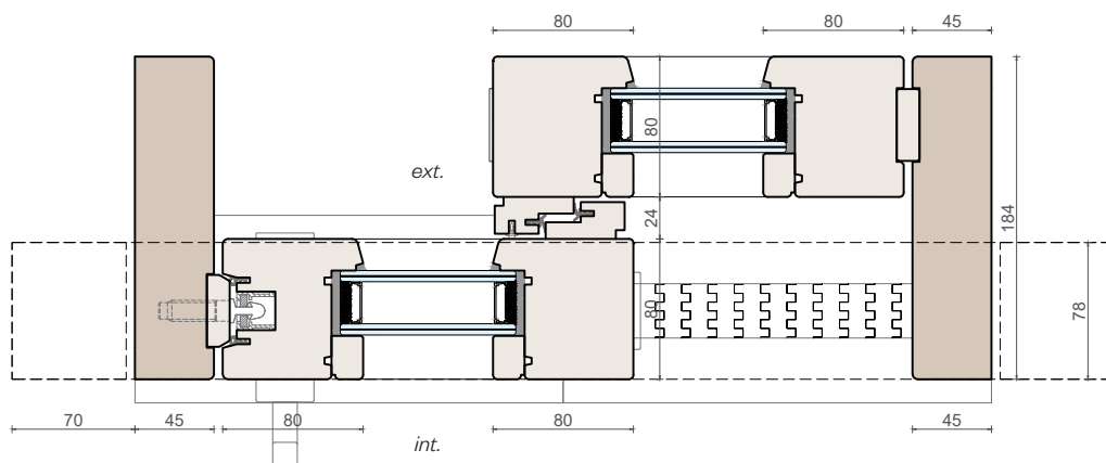
Sezione orizzontale
