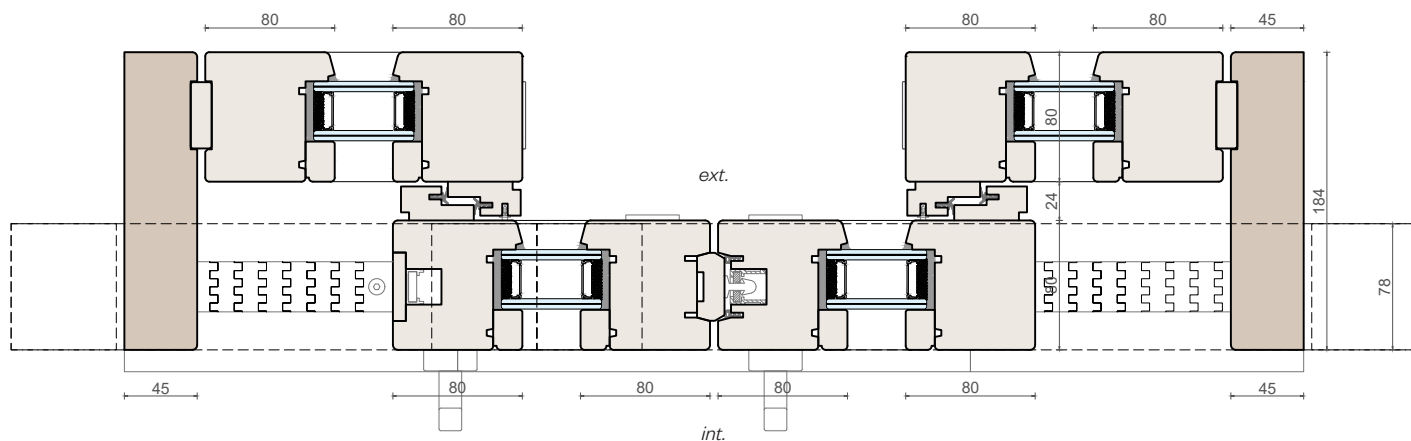
Sezione orizzontale
