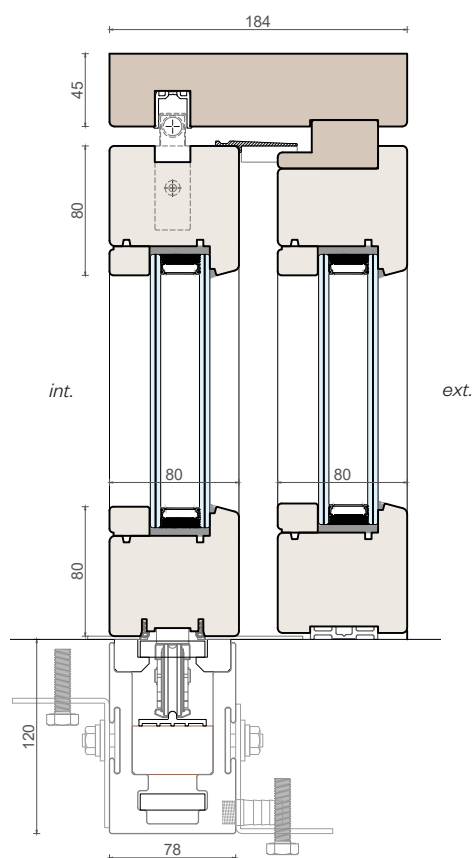
Sezione verticale
