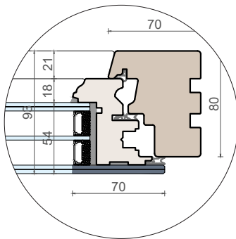
Fermavetro stile
