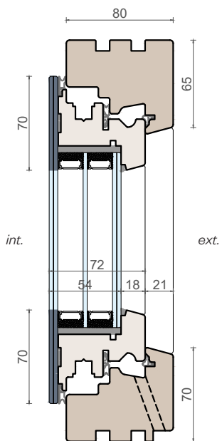
Sezione verticale
