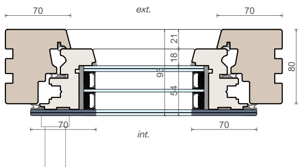
Sezione orizzontale
