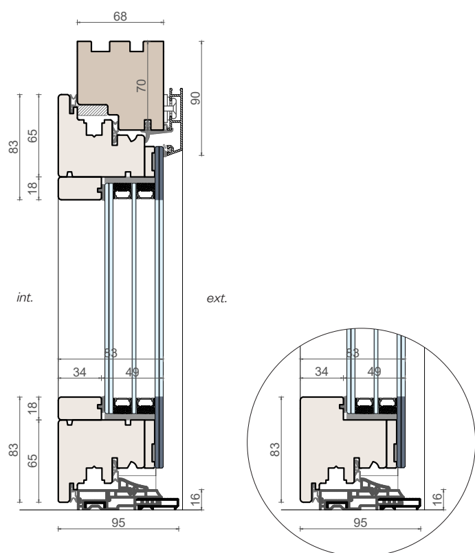
Sezione verticale
