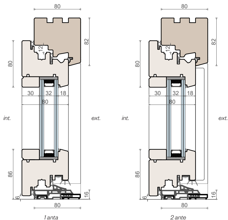
Sezione verticale
