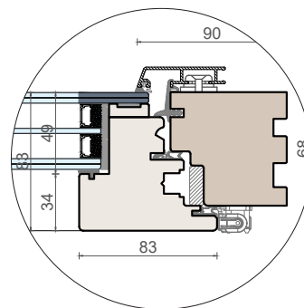
Fermavetro fisso
