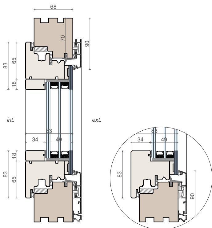
Sezione verticale
