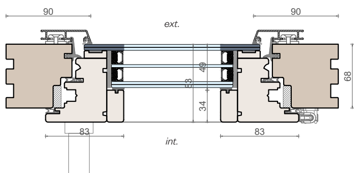
Sezione orizzontale
