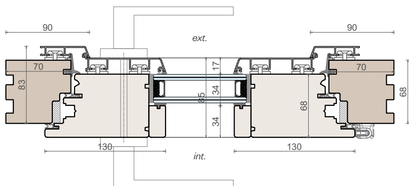
Sezione verticale
