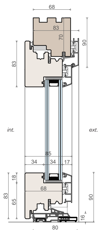
Sezione verticale
