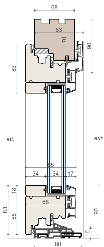
Sezione verticale
