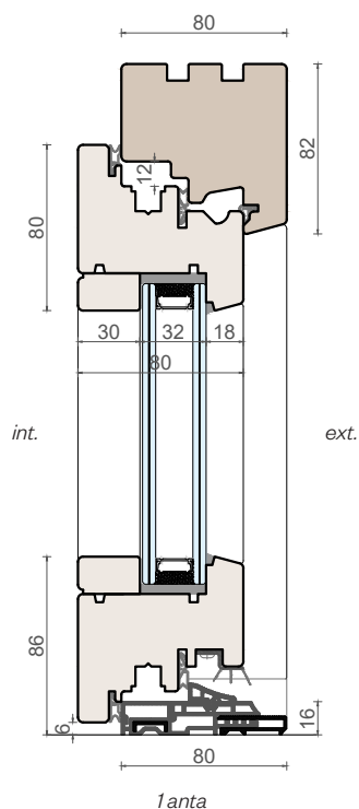
Sezione verticale
