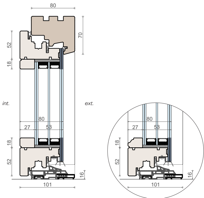
Sezione verticale
