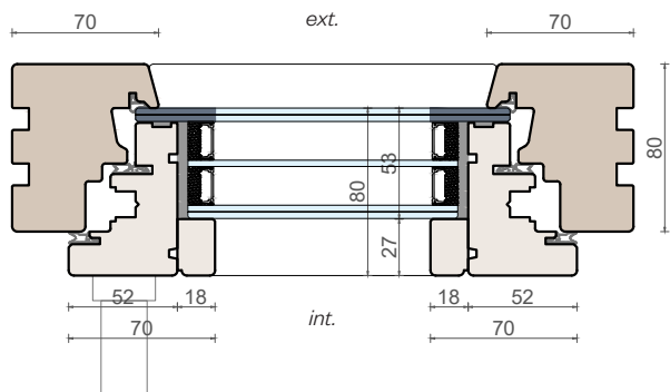
Sezione orizzontale
