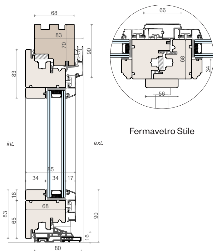
Sezione verticale
