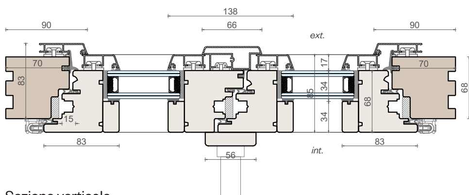
Sezione verticale
