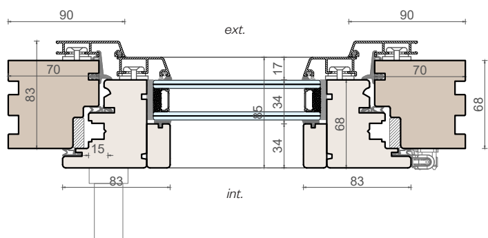
Sezione orizzontale
