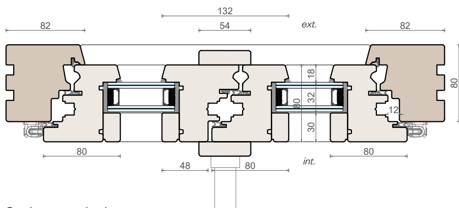
Sezione verticale
