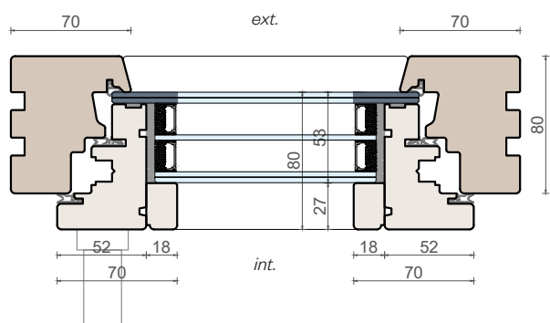
Sezione orizzontale
