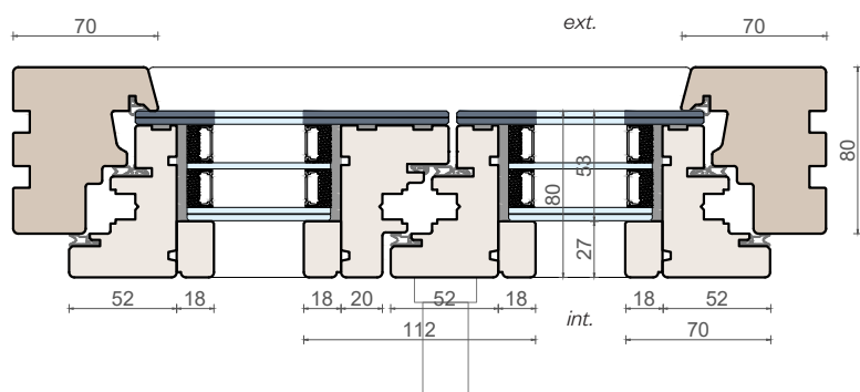
Sezione verticale
