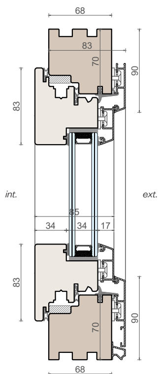
Sezione verticale Versione Quadra
