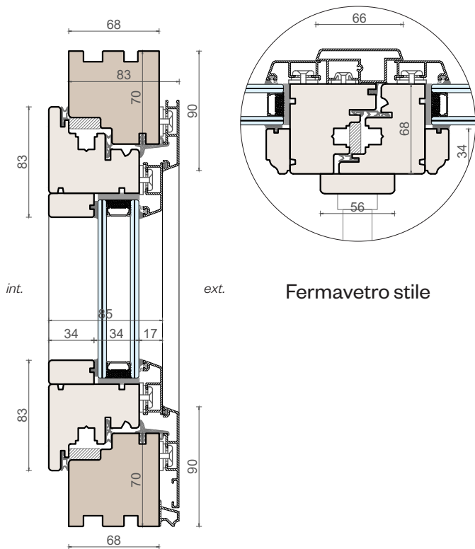
Sezione verticale
