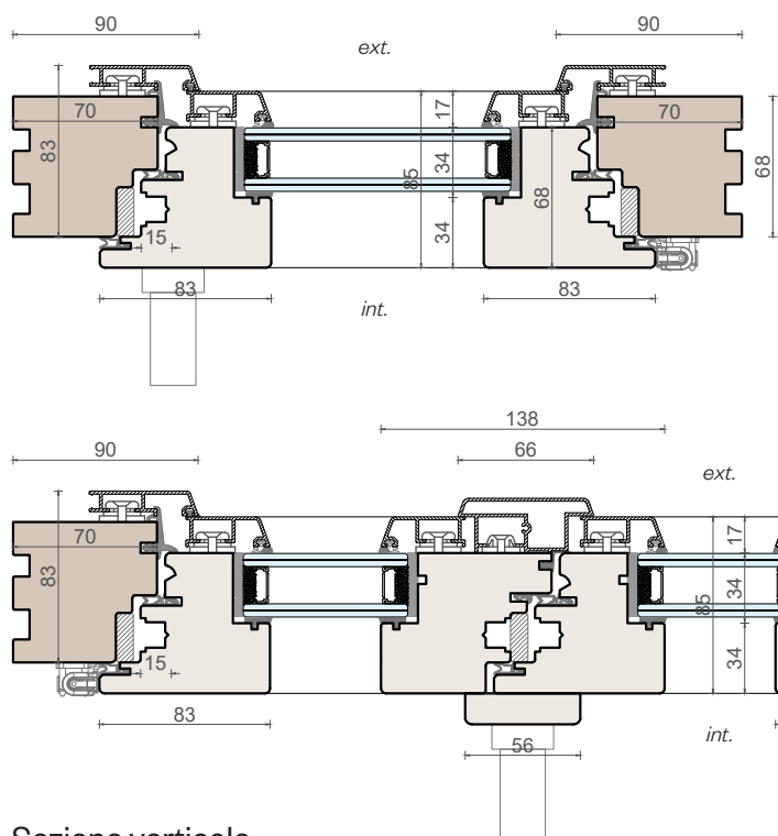
Sezione verticale Versione Quadra
