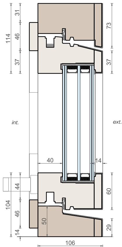
Sezione verticale
