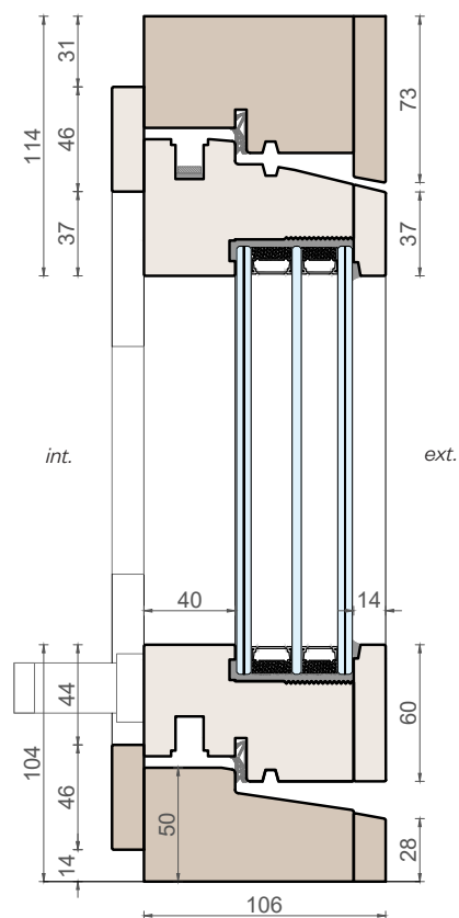
Sezione verticale
