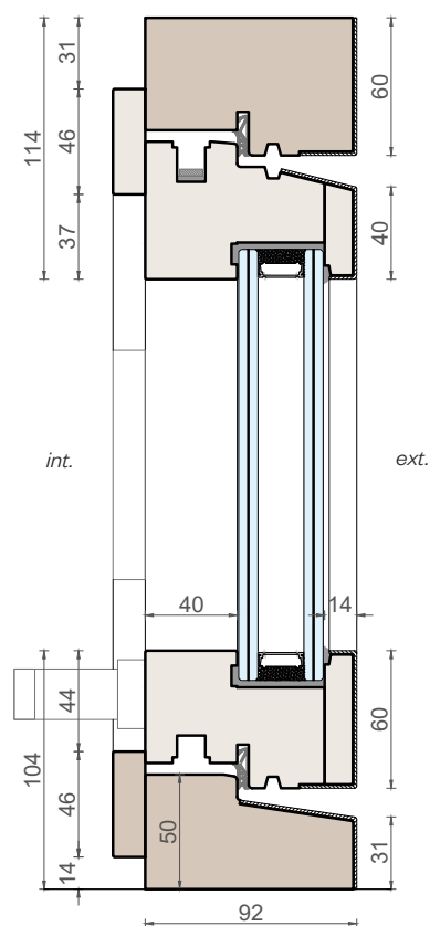
Sezione verticale
