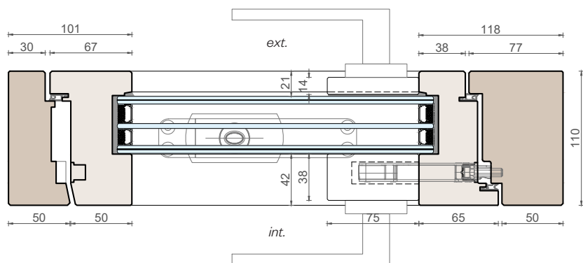
Sezione orizzontale
