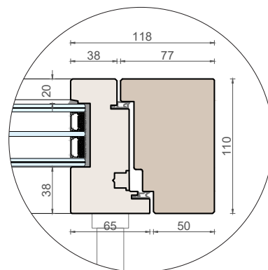
Massima sede vetro
