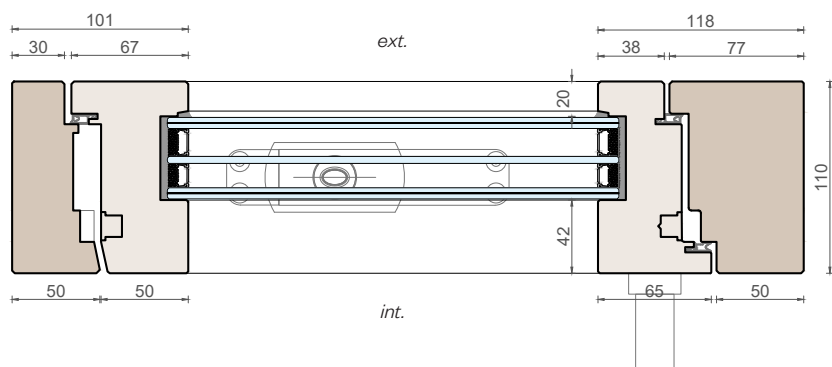
Sezione orizzontale
