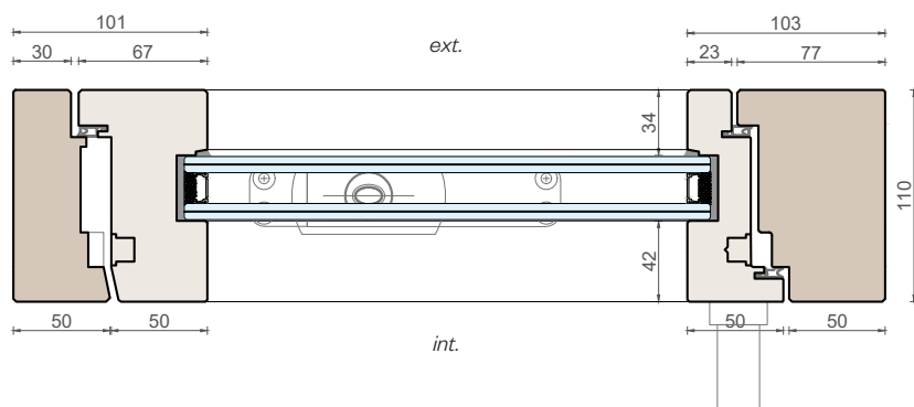
Sezione orizzontale
