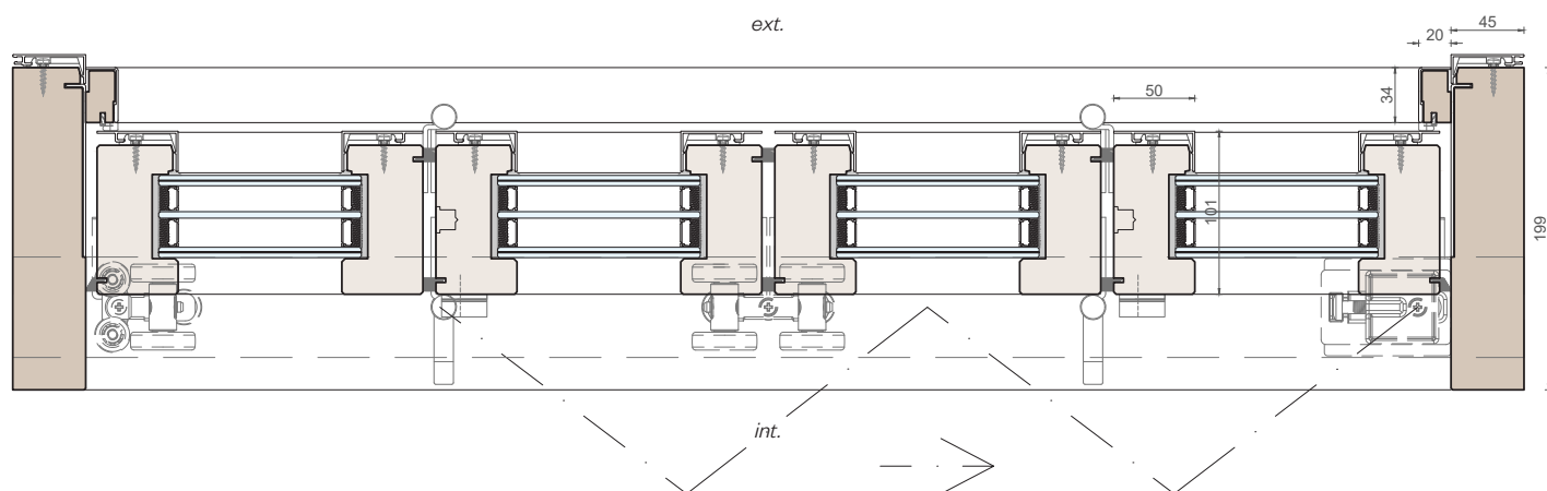
Sezione orizzontale
