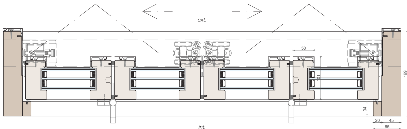
Sezione verticale
