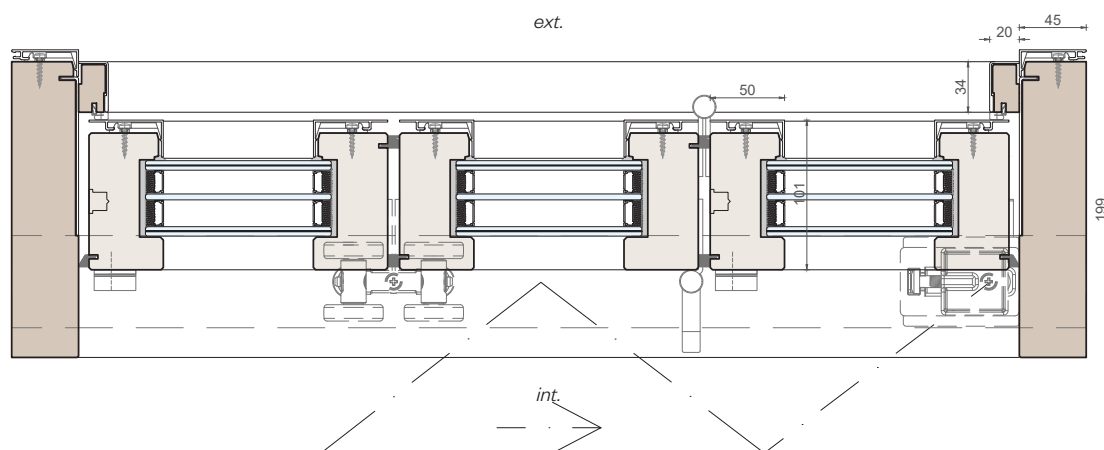
Sezione orizzontale
