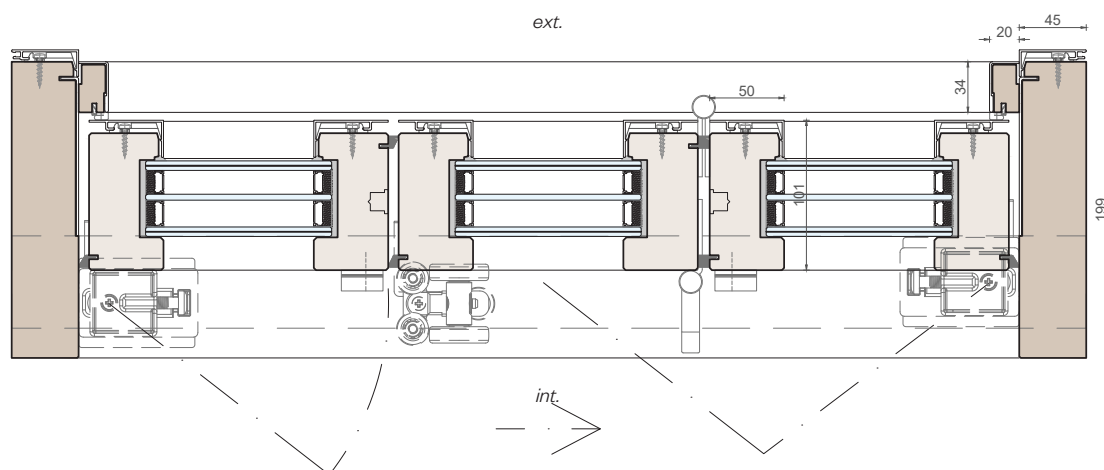
Sezione orizzontale
