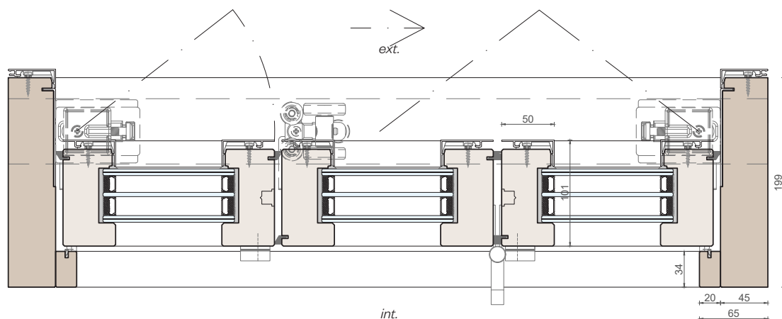
Sezione verticale
