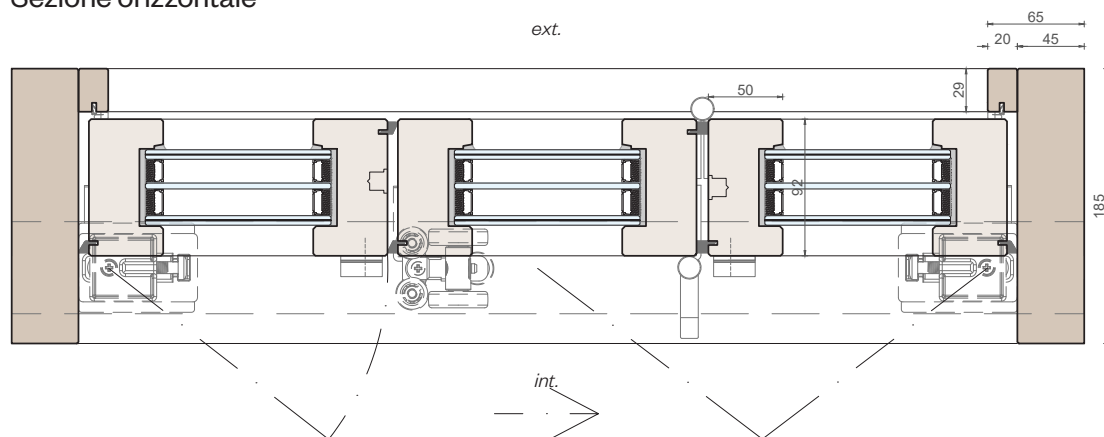
Sezione orizzontale
