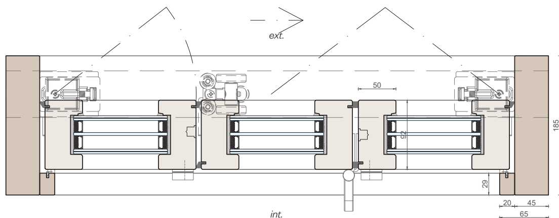
Sezione verticale
