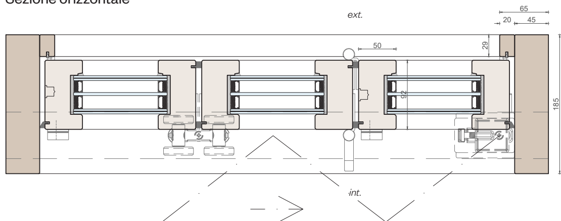
Sezione orizzontale
