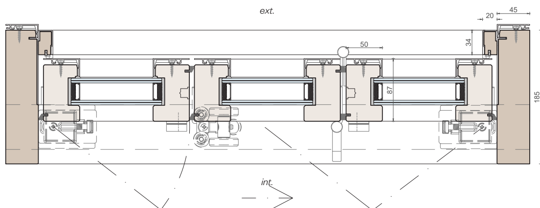
Sezione orizzontale
