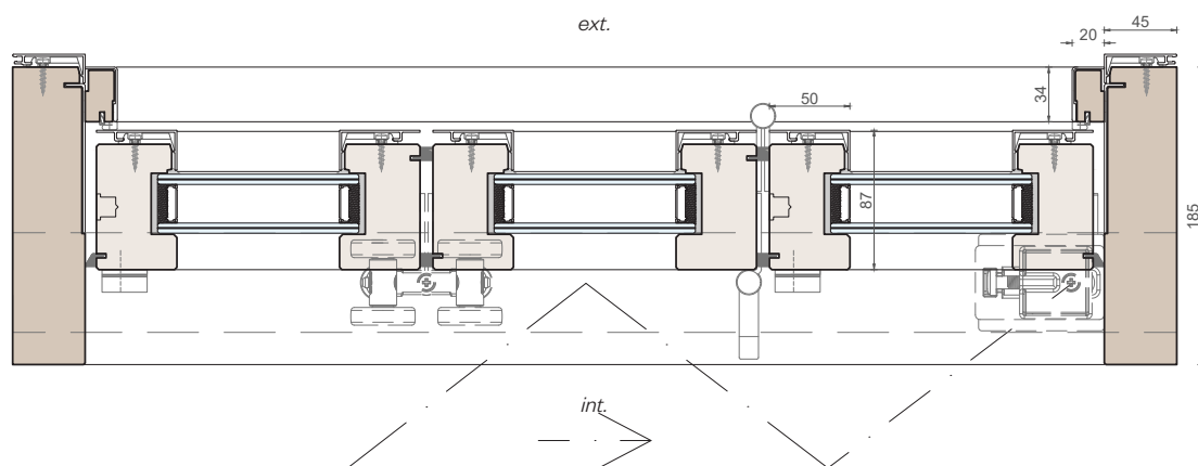
Sezione orizzontale
