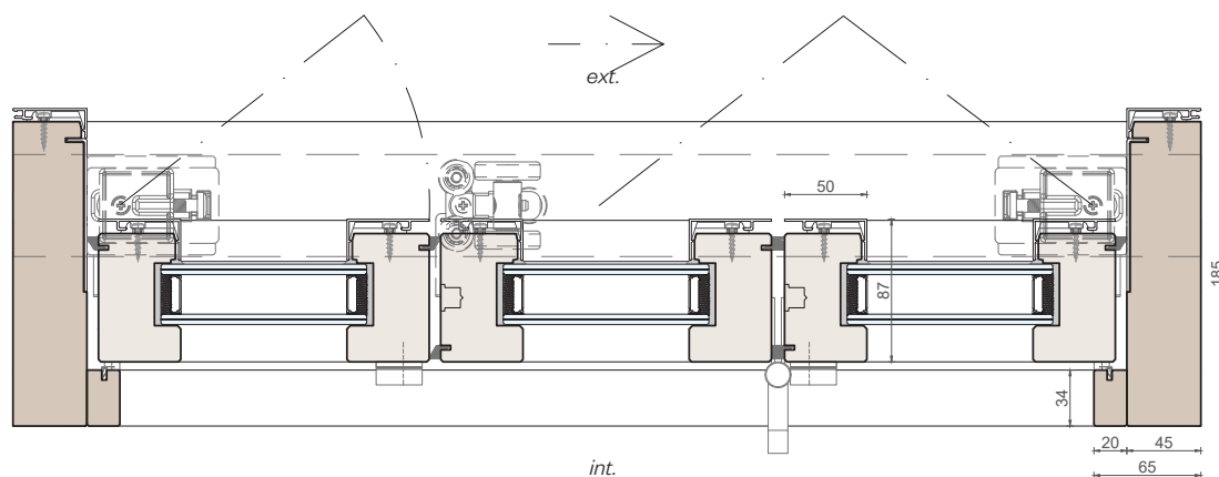
Sezione verticale
