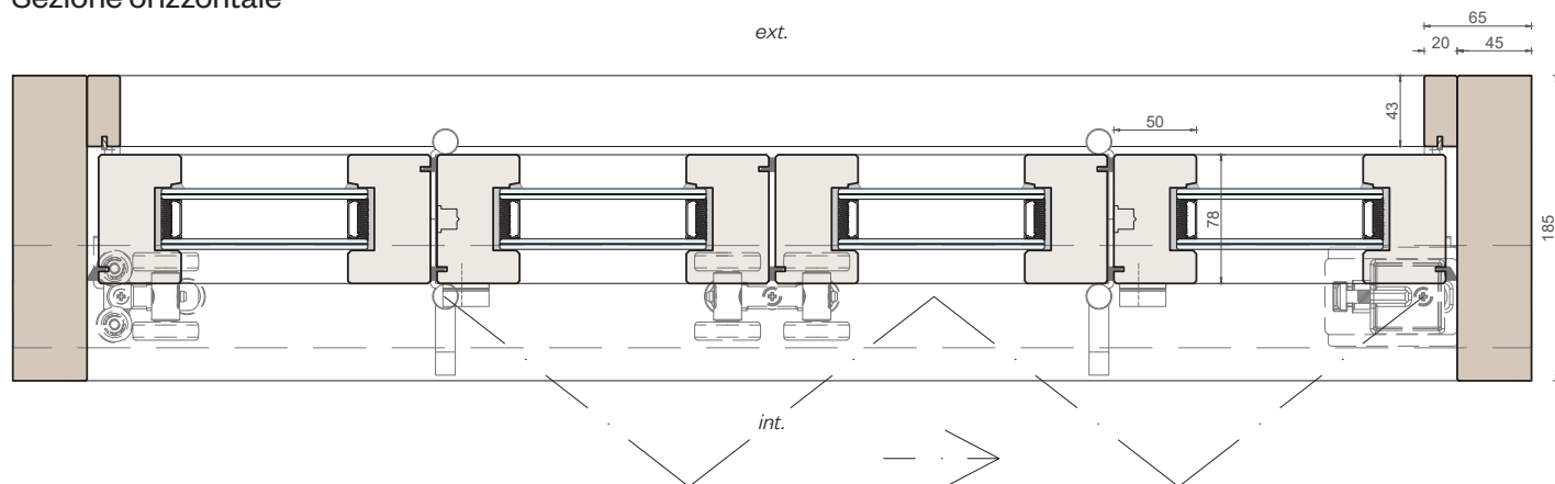
Sezione orizzontale
