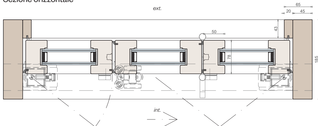
Sezione orizzontale
