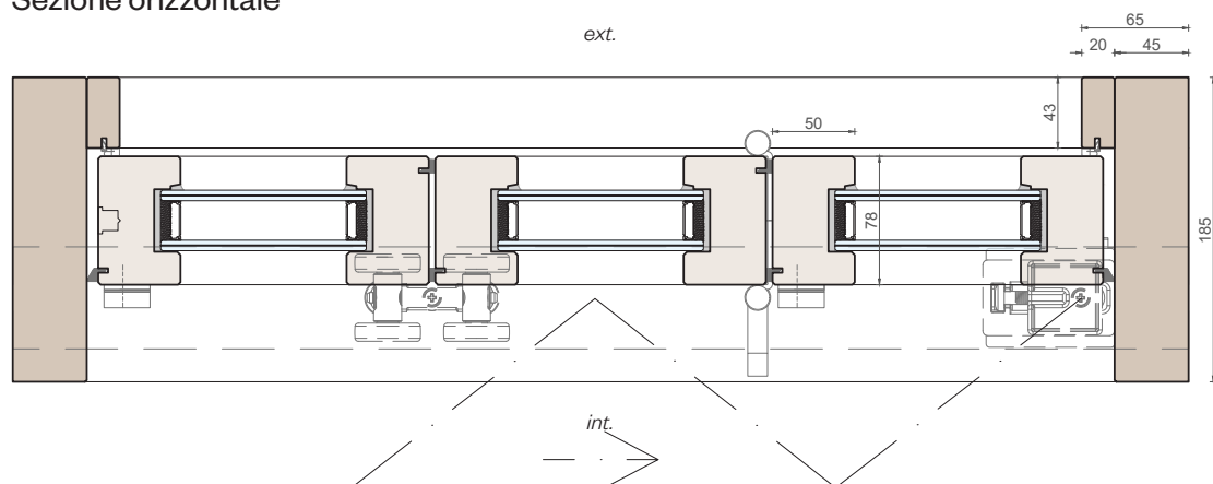
Sezione orizzontale
