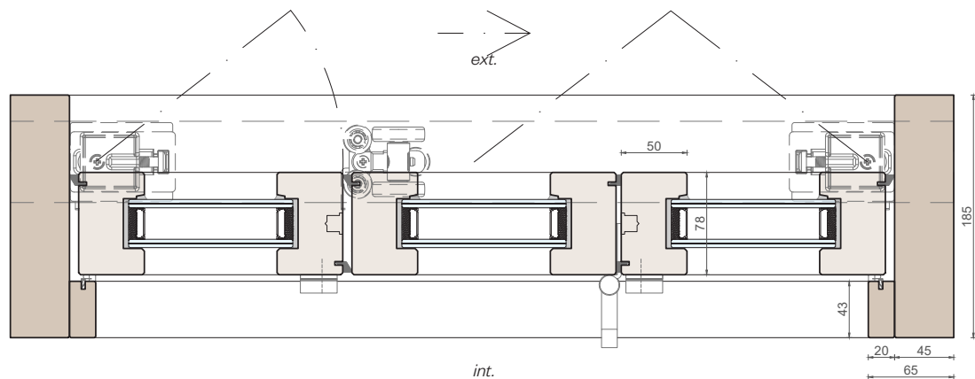
Sezione verticale
