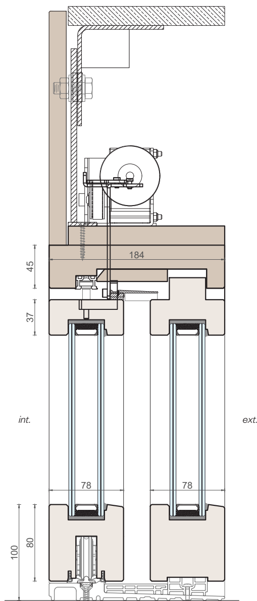
Sezione verticale
