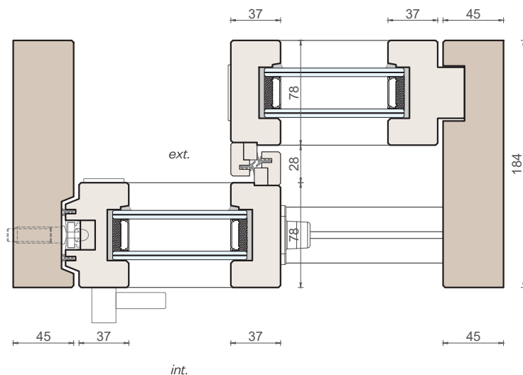
Sezione orizzontale
