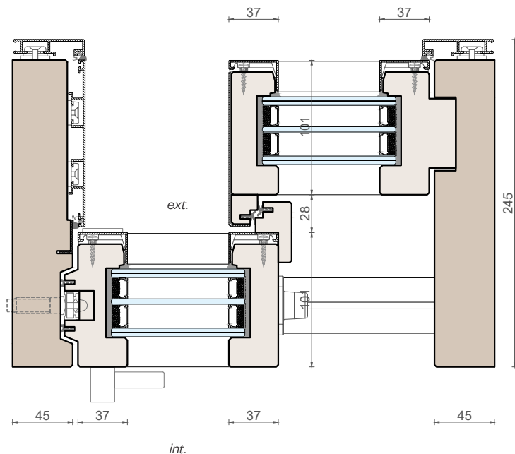
Sezione orizzontale
