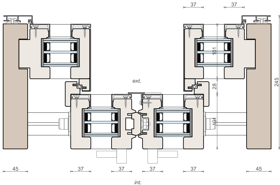
Sezione orizzontale
