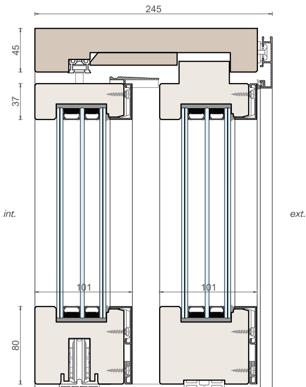
Sezione verticale
