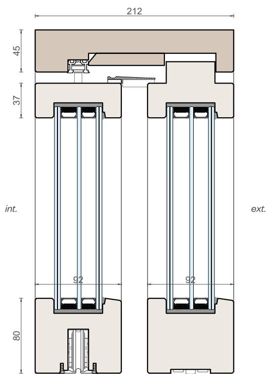
Sezione verticale
