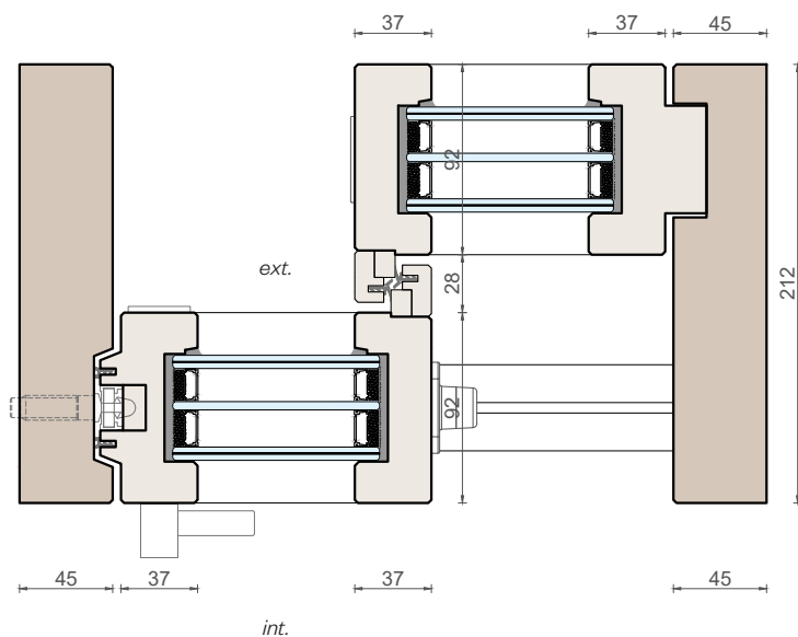
Sezione verticale
