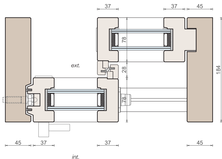
Sezione orizzontale
