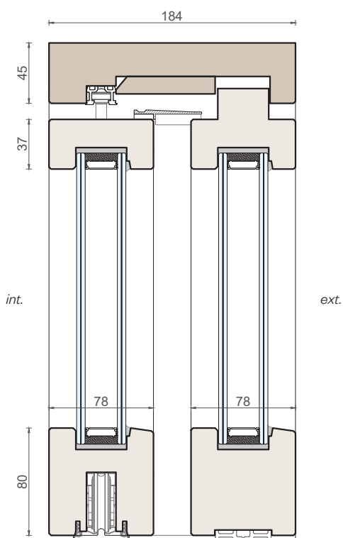
Sezione verticale
