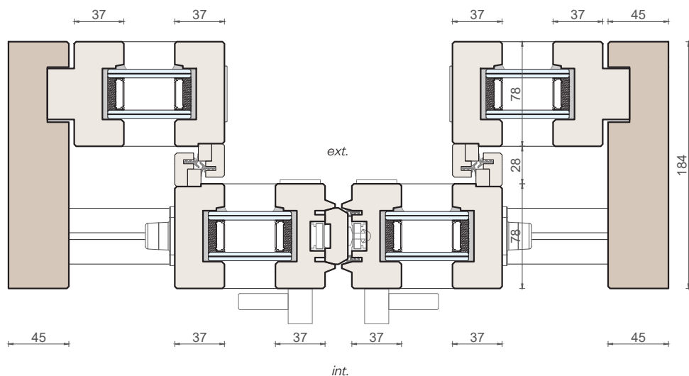
Sezione orizzontale
