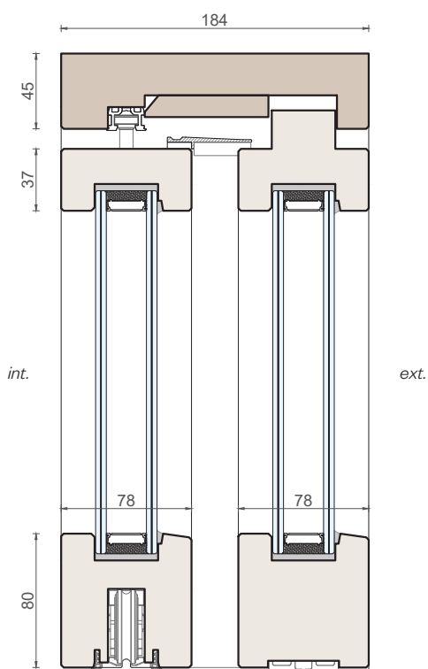
Sezione verticale
