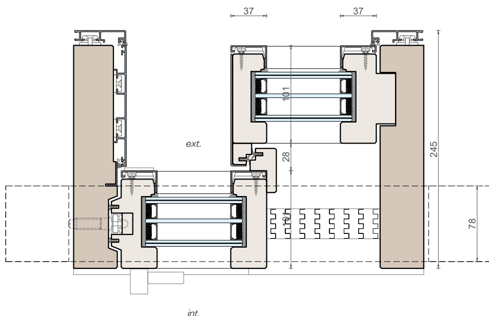
Sezione verticale
