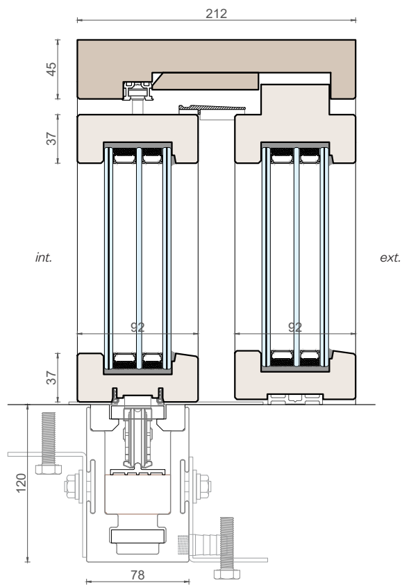
Sezione verticale
