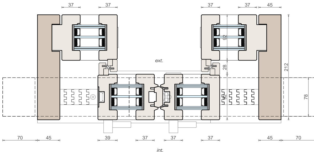
Sezione verticale
