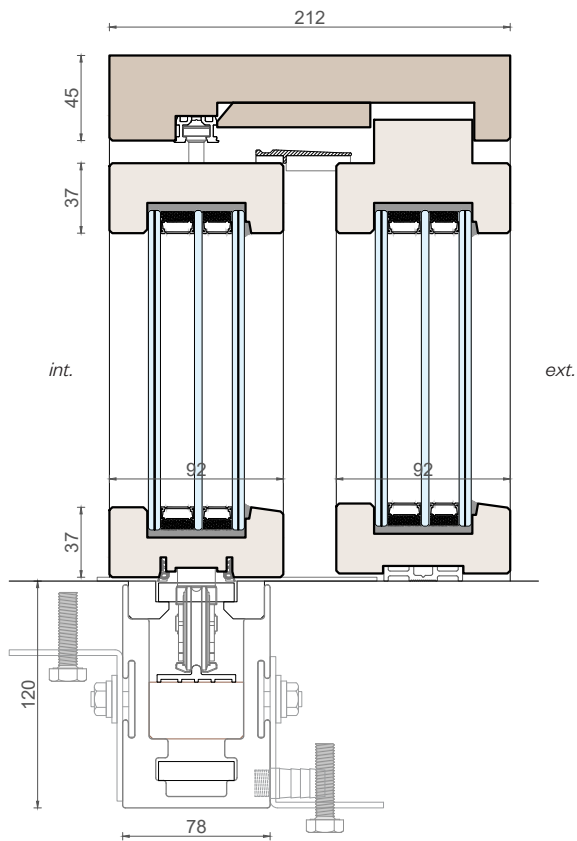
Sezione verticale
