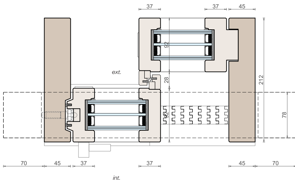
Sezione verticale
