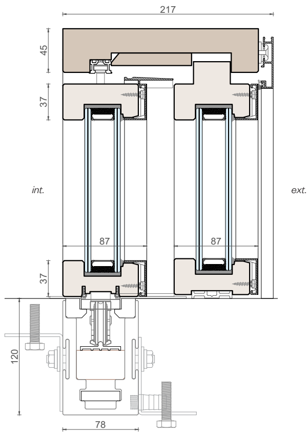
Sezione verticale
