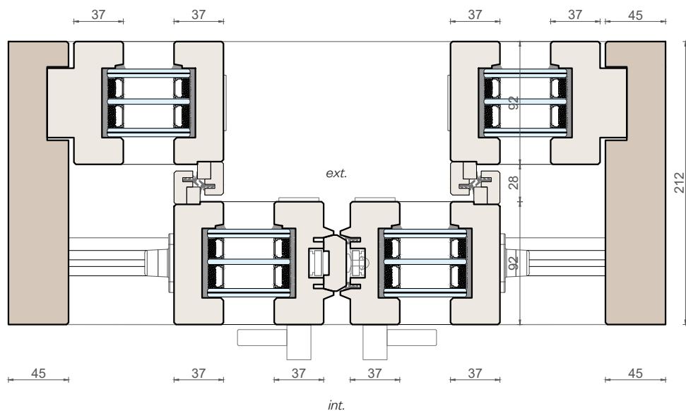
Sezione verticale
