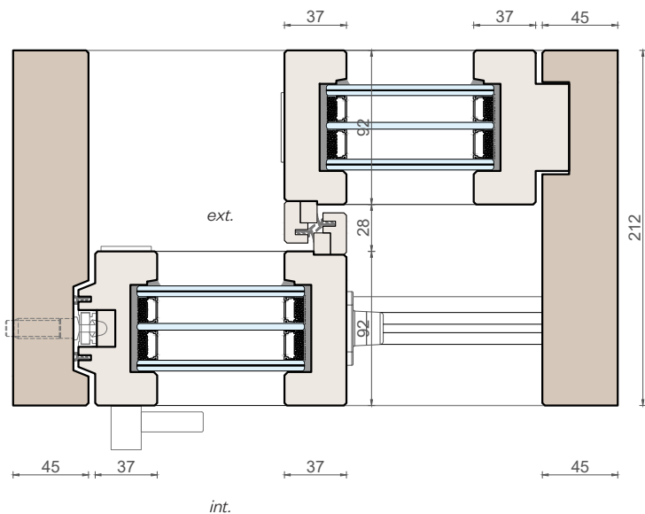
Sezione verticale
