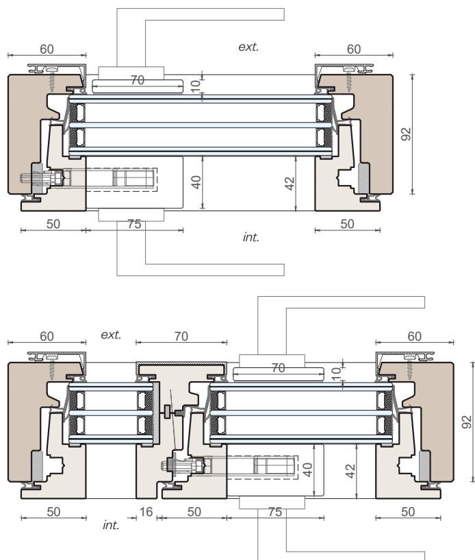
Sezione verticale
